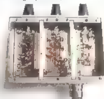
Triplexer voor groot vermogen (800 W HF/VHF, 300 W UHF, 150 W 5HE, vswr <math>\leq 1,2</math>)
